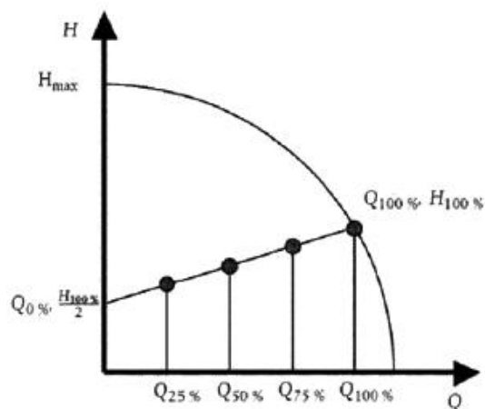
Рис.1. Опорная контрольная линия циркуляционного насоса
