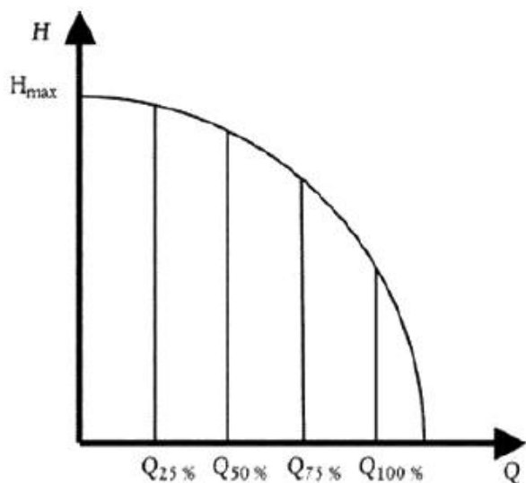
Рис.3. Профиль нагрузки
